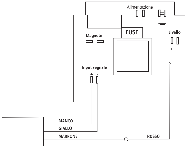
Fig. 39. Schema circuito VMS MF per la connessione ad un contatore lancia impulsi con effetto Hall
