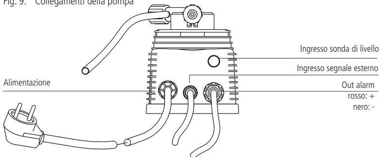
Fig. 9. Collegamenti della pompa
